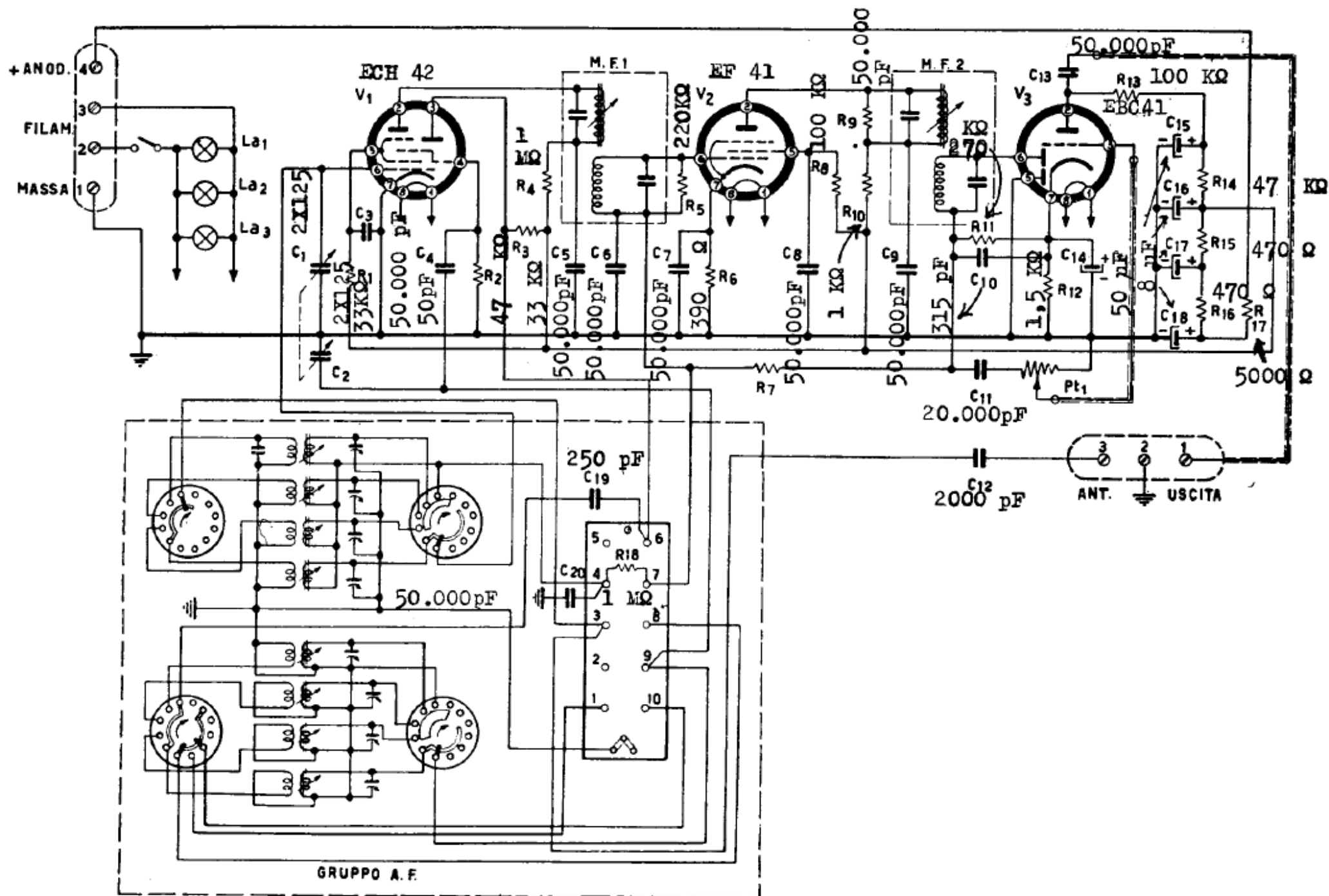
LESAs - RADIOSINTONIZZATORE mod. RS/3. Gruppo AF Dm 12249. Trasformatore MF 1° stadio Dm 12250. Trasformatore MF 2° stadio Dm 12250/1. Nel caso di alimentazione con il preamplificatore tipo PR/10 o PR/20, sostituire la R17 da 5000 Ω 4 watt con una resistenza da 470 Ω 1 watt.
